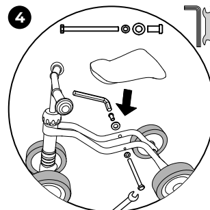
Sædet anbringes på rammen og skrues fast
