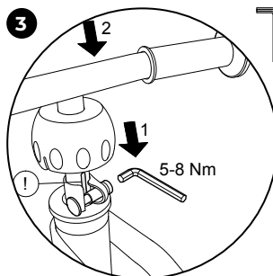
Styr skydes til anslag på gaffel og skruen spændes. Slids i styrpind rettes bagud(!). Kugle trykkes herefter fast nedad indtil den falder i hak.
