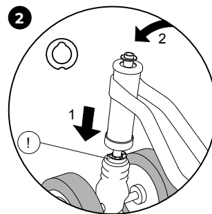
Gaffel skydes på styrehovedrør, til anslag. Korrekt justering af styreleje observeres(!). Underlagsskive monteres.
